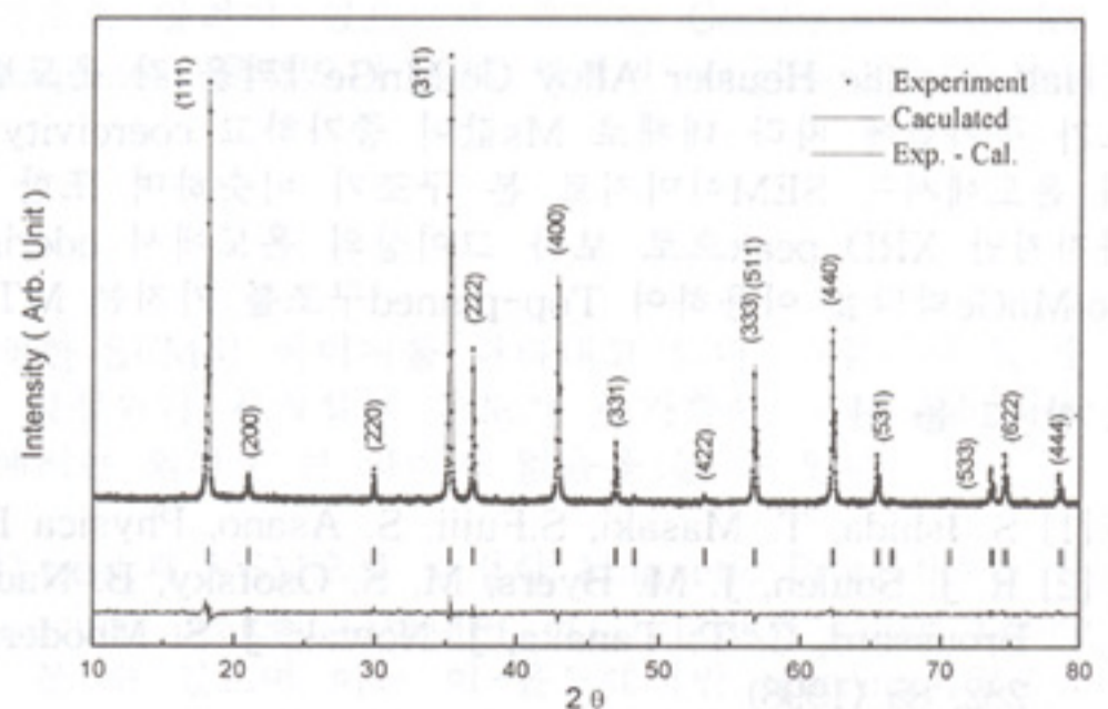
그림. 1 \text{Li}_{0.5}\text{Fe}_{1.0}\text{Rh}_{1.5}\text{O}_4 의 X-선 회절도
