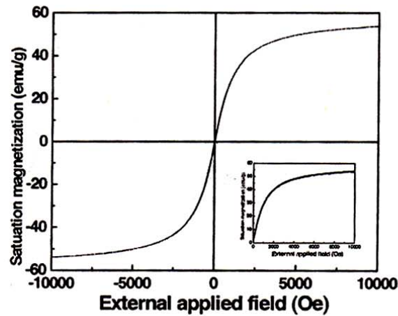
Fig. 2. MgFe_2O_4 나노입자의 자기이력곡선
