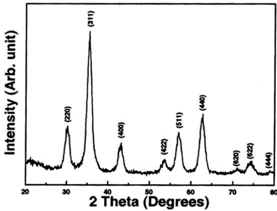
Fig. 1. MgFe_2O_4 나노입자의 X-선 회절도
