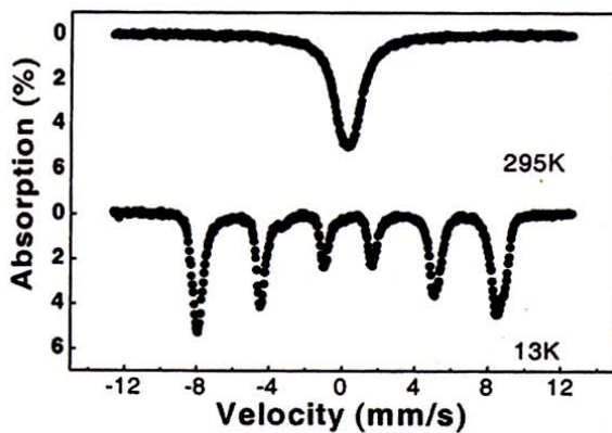
Fig. 3. MgFe_2O_4 나노입자의 Mössbauer Spectrum
