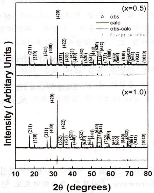
Fig. 1. \text{Tb}_{3-x}\text{Bi}_x\text{Fe}_5\text{O}_{12} 의 X-선 회절도
