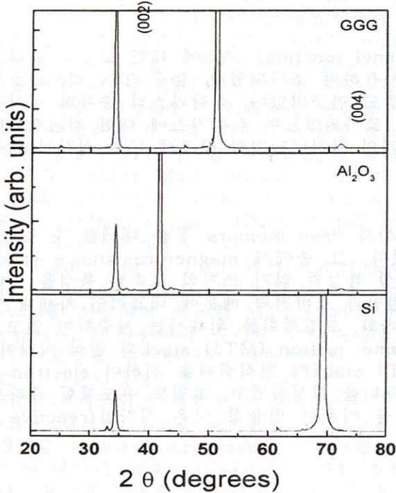
Fig. 1 기판에 따른 Zn 0.97 Fe 0.03 O 박막의 X-선 회절도 (T sub. = 500 °C)
